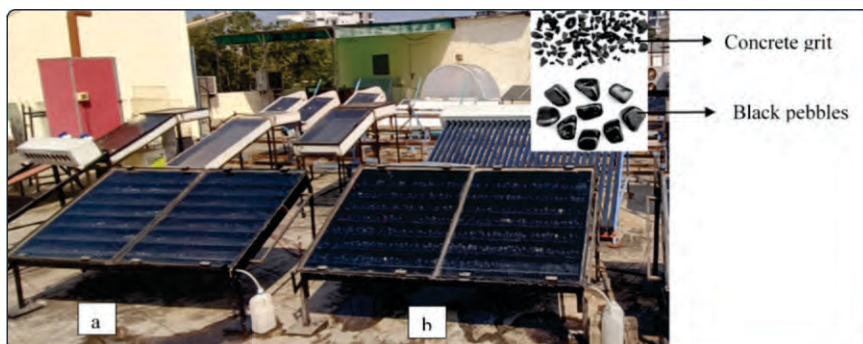
चित्र: प्रायोगिक सेटअप। सौर स्टिल के फोटोग्राफ (a) कंक्रीट गिट के साथ, (b) ब्लैक कंकड़ के साथ Figure: Experimental setup. Photographs of solar still with (a) concrete grit, (b) black pebble
