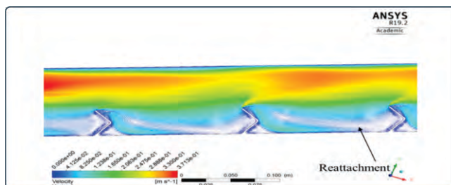
चित्र: सौर संग्राहक पर कृत्रिम प्रवर्धकों के सीएफडी अध्ययन Figure: CFD studies of artificial enhancers on solar collector
