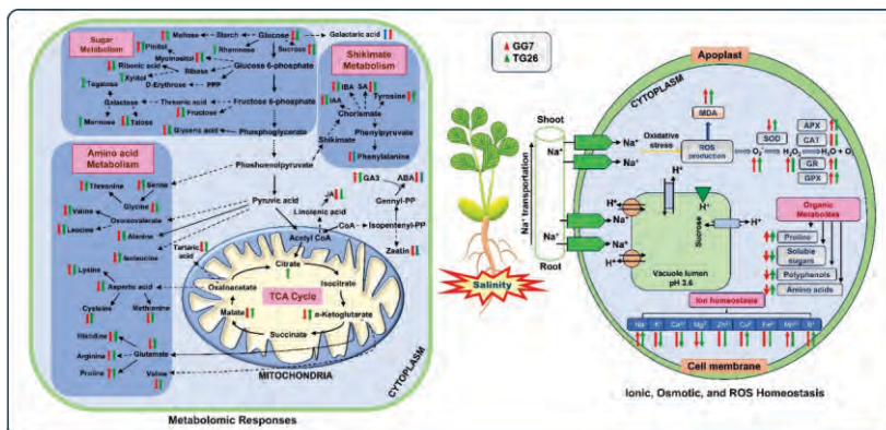
चित्र: अरचिस हाइपोगेआ में लवणता सहिष्णुता तंत्र का योजनाबद्ध प्रतिनिधित्व Figure: Schematic representation of salinity tolerance mechanisms in Arachis hypogaea
